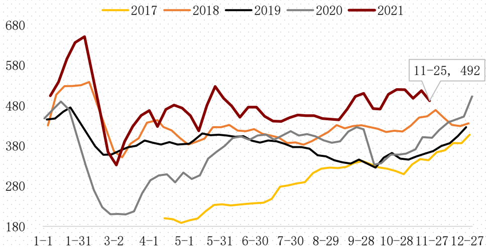
49家短流程废钢库存（万吨）
