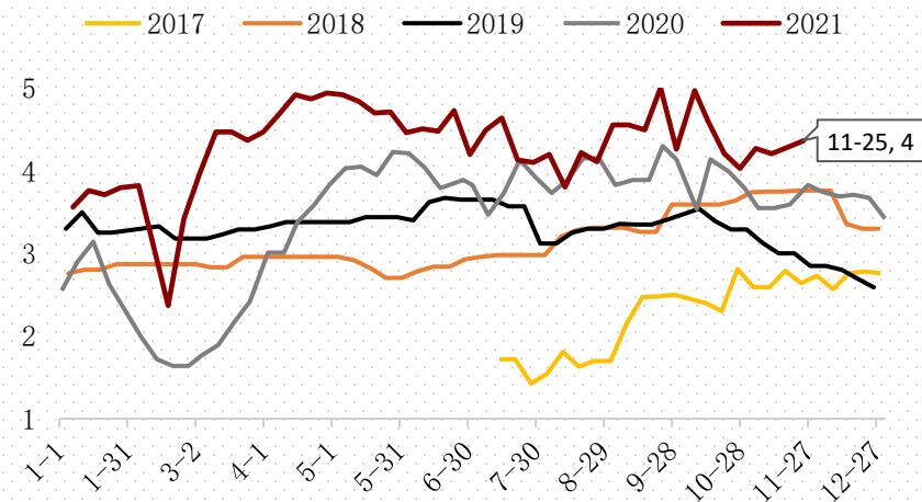
华中钢厂废钢日耗(万吨)
