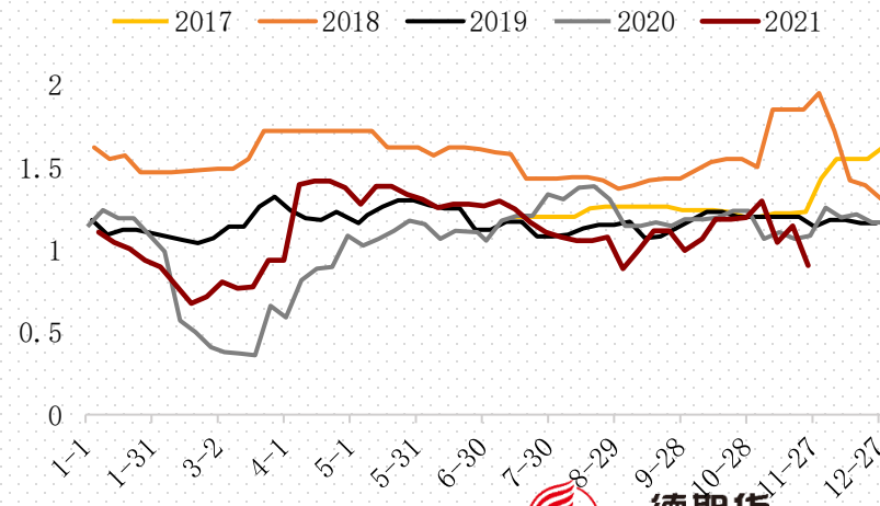
辽宁废钢日耗 (万吨)
