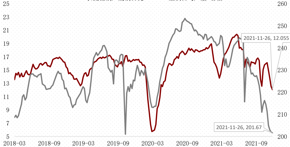
生铁日均产量和废钢日耗（万吨）
