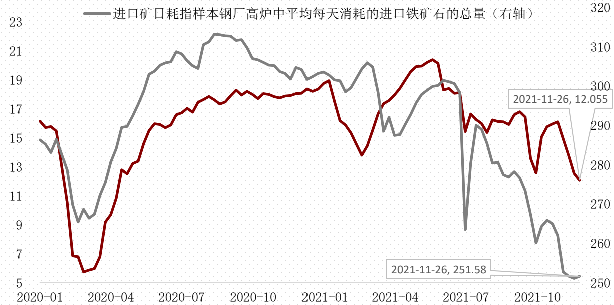
长流程废钢日耗和进口矿日耗对比（万吨）
