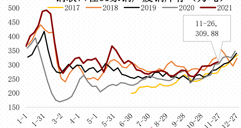
钢联口径61家钢厂废钢库存（万吨）
