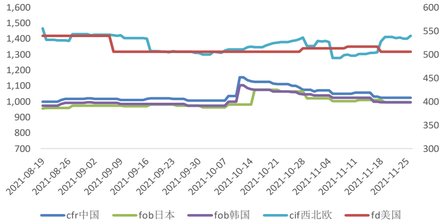
丙烯
