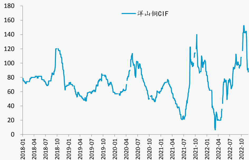
图3：洋山铜溢价
