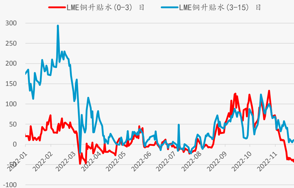
图4：伦铜升贴水
